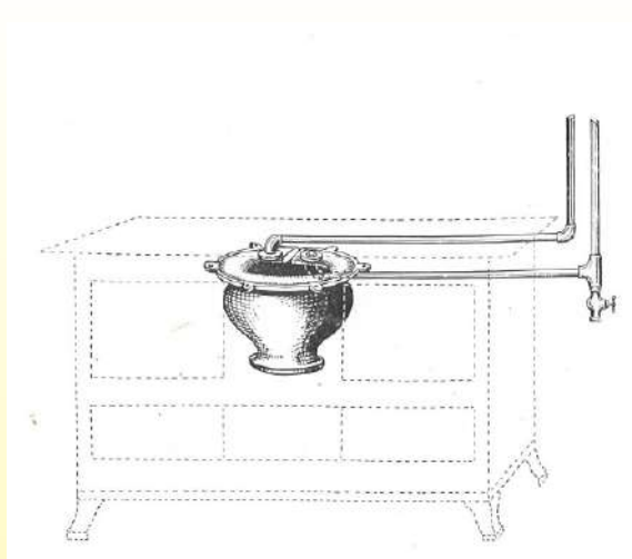
Scambiatore di calore "Bouilleur" montato all'interno di una stufa (Catalog of Ets Demoulin, Farcienne, 1932, Ultimheat Museum)
